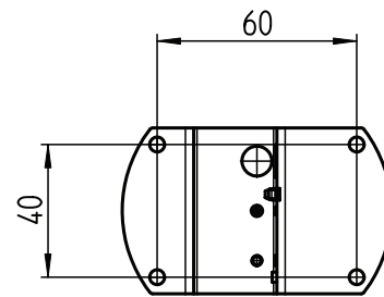
Ansicht ohne Abdeckung
