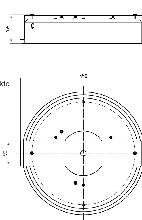
Variante Einbaubügel
