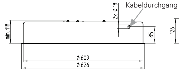
Variante Direkt
