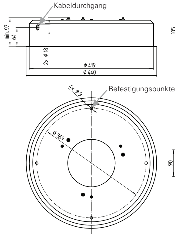
Variante Direkt
