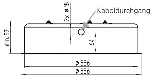
Variante Direkt
