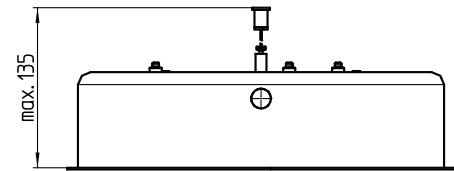
Variante Pendel
