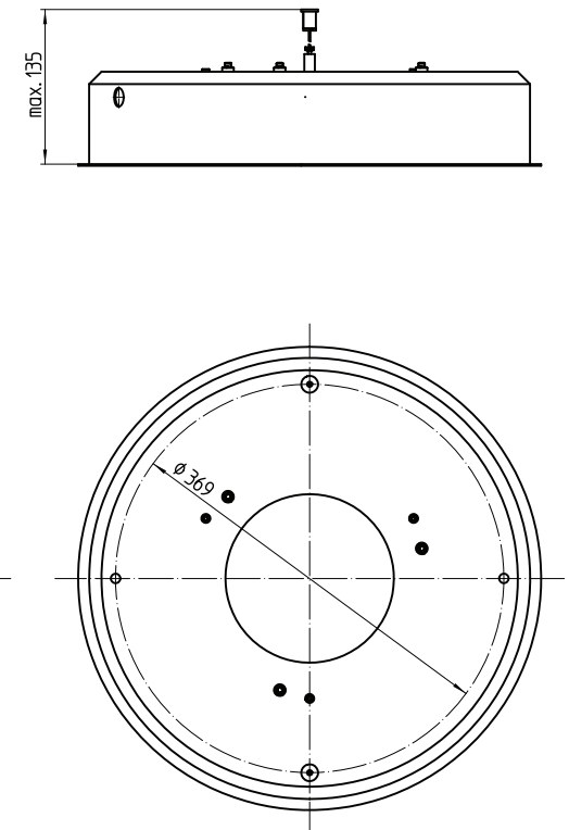
Variante Pendel
